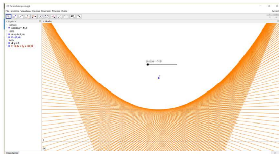
Figura 8. Costruzione della parabola come inviluppo delle tangenti su GeoGebra
