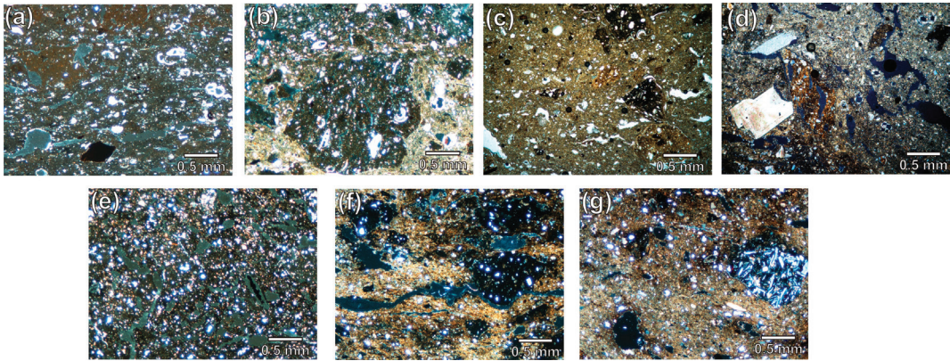
Figure 5. Thin sections of the specimens belonging to the five fabrics identified. Fabric Ch MC : (a) OG12/140, (b) CAN71/94, (c) BN7; Fabric CC MC : (d) BN23; Fabric Ch QF : (e) 18704; Fabric Ch FM : OG12/154 (f) ; Fabric Ch VM : OG12/6 (g).
