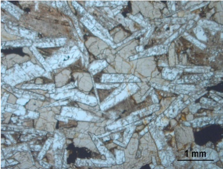
Fig. 14. Dolerite caratterizzata da una tessitura subofitica definita da plagioclasio idiomorfo incluso in cliopirosseno interstiziale. sezione 65, immagine al microscopio ottico, solo pol.
