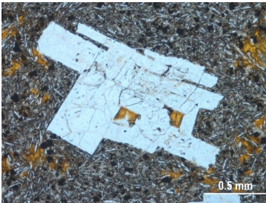
Fig. 11: Glomerofiro di plagioclasio inglobato in una massa di fondo pilotassitica. Sezione 71, immagine al microscopio ottico, pol. X.
