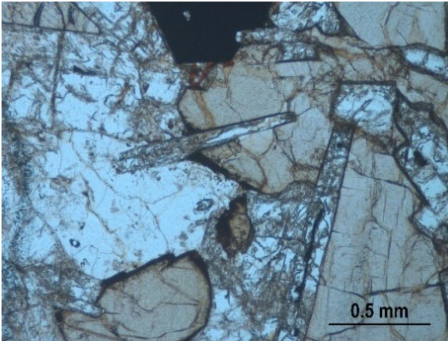
Fig. 15. Dettaglio di leucite in associazione con clinopirosseno. Sezione 67, immagine al microscopio ottico, solo pol.
