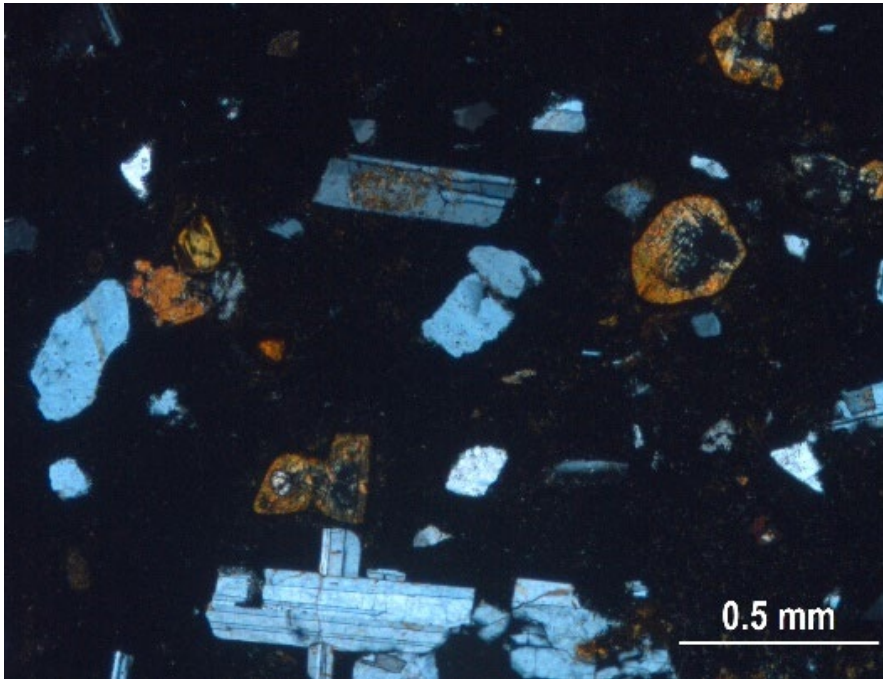
Fig. 10: Tessitura porfirica con fenocristalli di plagioclasio e olivina immersi in una massa di fondo vetrosa. Sezione 66, immagine al microscopio ottico, pol. X.
