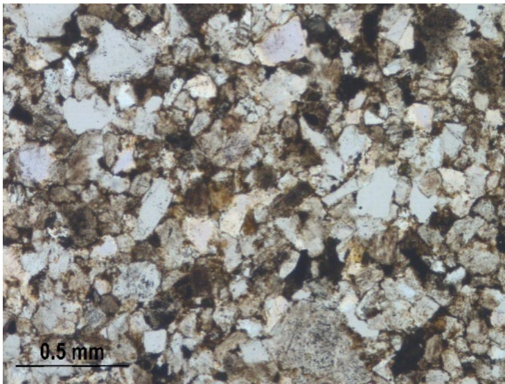
Fig. 5: Arenaria mal classata. Si osservano clasti poco arrotondati di quarzo prevalente in un cemento siliceo. Sezione n°11, microscopio ottico, nicol paralleli.
