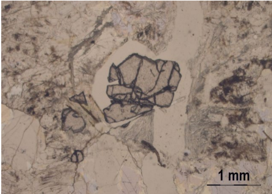
Fig. 7: (a) Granulite acida. Campione 36, costituito da 3 frammenti, ed un foglietto in cui si attesta la provenienza da un "granito" a cui era associato lo stesso numero di catalogo. Fig. 8: sezione n. 6, associazione di alto grado metamorfico a granato e sillimanite. Immagine al microscopio ottico, solo pol.
