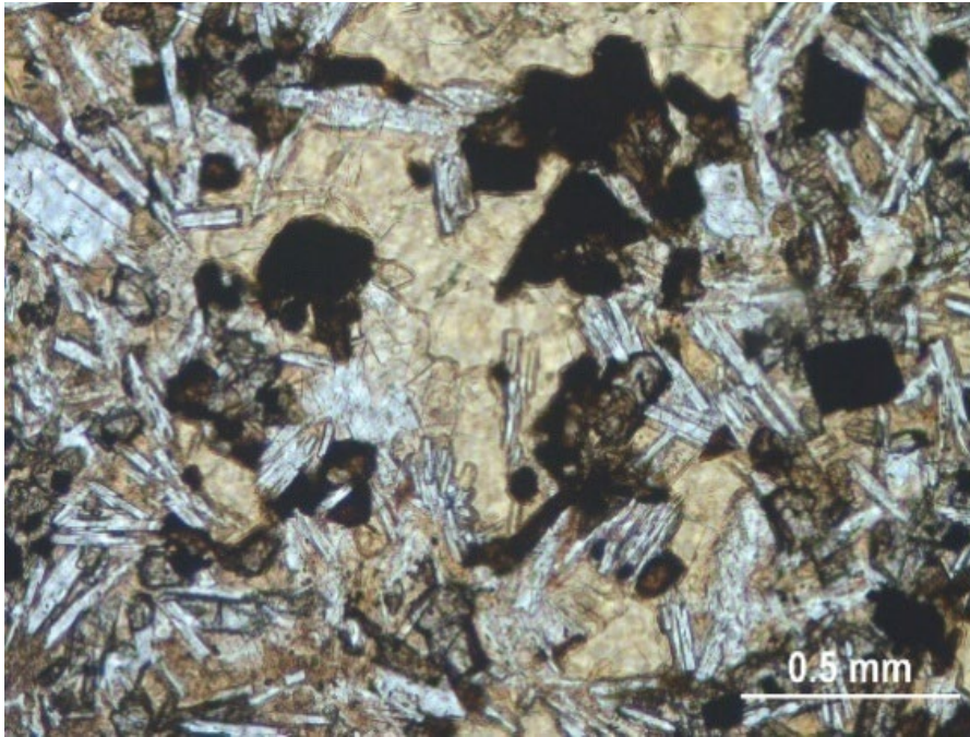
Fig. 13: Palagonite intersertale nella massa di fondo. Sezione 71, immagine al microscopio ottico, solo pol.
