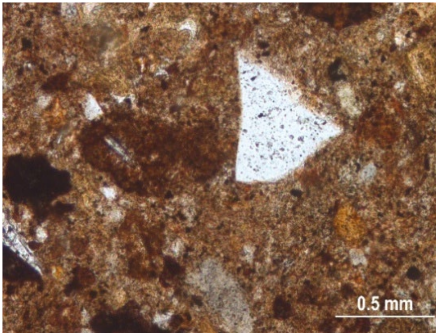
Fig. 6: Grovacca con clasto spigoloso di quarzo in una matrice pelitica. Sezione n°79, microscopio ottico, nicol paralleli
