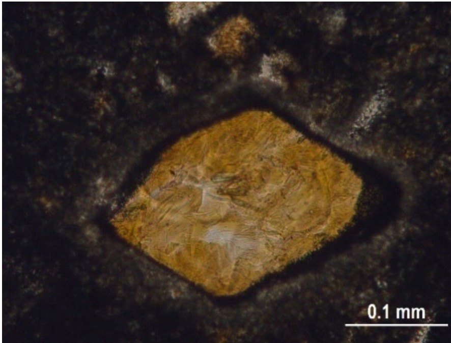
Fig. 12: Basale di Olivina alterata in bowlingite con massa di fondo cripto cristallina. Sezione 66, immagine al microscopio ottico, pol. X.
