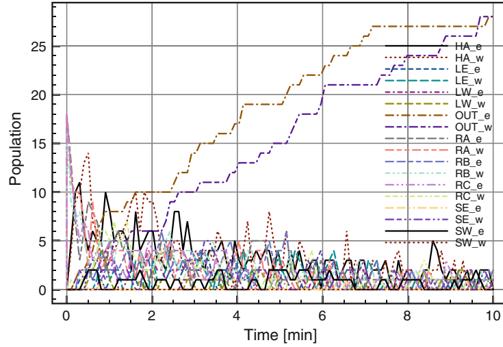
(b) Bio-PEPA: Arrivals (ODE)
