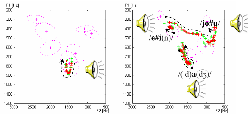
Figura 19. Diagrammi Voweltrack : (a) dell'incontro vocalico del passaggio in Fig. 18; (b) degl'incontri vocalici e d'una vocale tonica del passaggio in Fig. 20.
