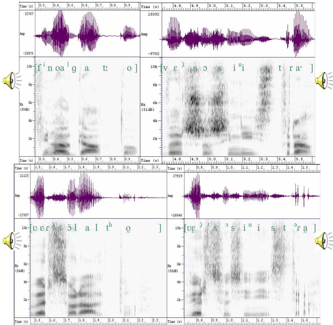
Figura 10. Realizzazioni di vocali atone finali prepausali a Bari (in alto, loc. p2M) e a Lecce (in basso, loc. p2M). In alto a sinistra: "fino al gatto" (Bmp2#22); in alto a destra: "verso sinistra" (Bmp2#82). In basso a sinistra: "verso l'alto" (Ltp2#208); in basso a destra: "verso sinistra" (Ltp2#56).
