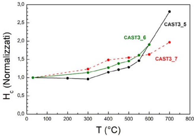
Fig. 192. Monitoraggio della variazione della suscettività magnetica durante la smagnetizzazione termica per diversi campioni del forno Cast 3.
