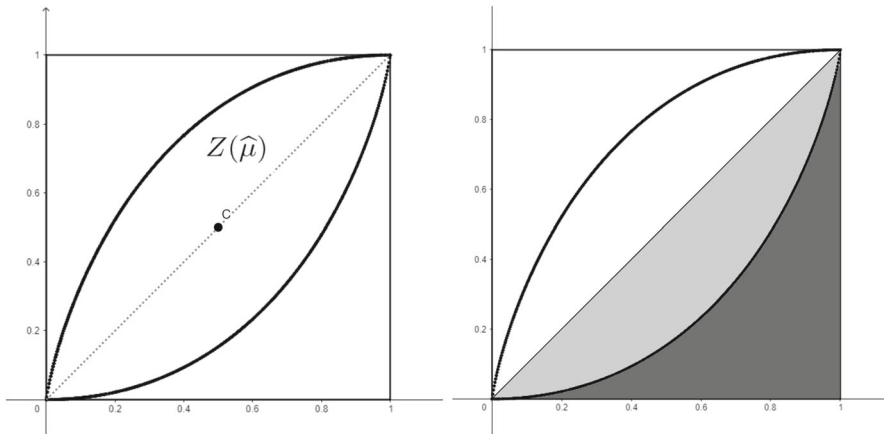
Fig. 2 Lorenz curve
