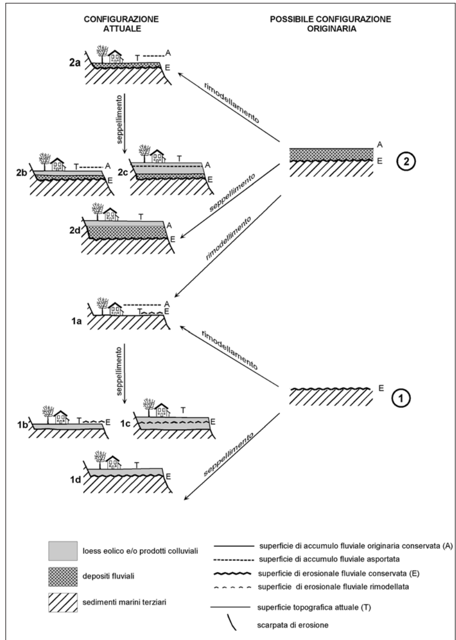
Fig. 7 - Diverse configurazioni ( T ) degli attuali lembi di superfici terrazzate ( 1a, 1b, 1c, 1d, 2a, 2b, 2c, 2d ) a partire dalle due possibili tipologie iniziali ( 1 e 2 ), a seguito di fenomeni di rimodellamento e/o seppellimento.
