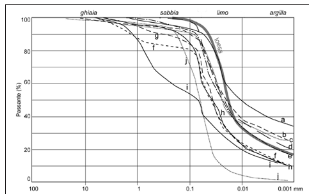
Fig. 6 - Curve granulometriche cumulative dei sedimenti presi in esame, confrontate con la curva del loess eolico affiorante a Villa Gualino: (a) Scuola di S. Margherita; (b) NE di Tetti Rovei; (c) Cavoretto; (d) Il Bellardo; (e) Villa S. Croce; (f) Villa Sambuelli; (g) Villa Rey; (h) E di Residenza Superga; (i) Torre; (j) Boccia d'Oro.
