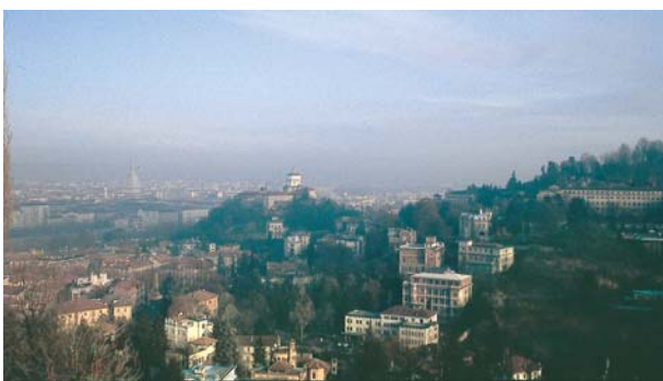
Fig. 10 - La sella in contropendenza che separa il lembo terrazzato del Monte dei Cappuccini dal resto del rilievo, connessa con l'incisione fluviale riferibile all'Unità 1, suggerisce che il sollevamento della Collina di Torino e la migrazione del suo margine settentrionale determinino il progressivo inglobamento nel rilievo di settori inizialmente di pianura.
