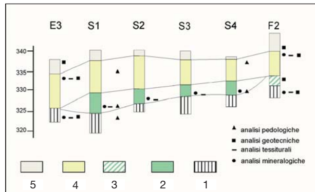
Fig. 2 - Il profilo geologico in corrispondenza al lembo di Villa Gualino (Unità 4 in Tav. 1) evidenzia un corpo sedimentario fluviale sviluppato in discordanza al di sopra del substrato marino e coperto dal loess eolico. 1) substrato marino; 2) depositi fluviali; 3) depositi colluviali; 4) loess eolico; 5) terreno di riporto (modificato da BOANO et al. , 2004).
