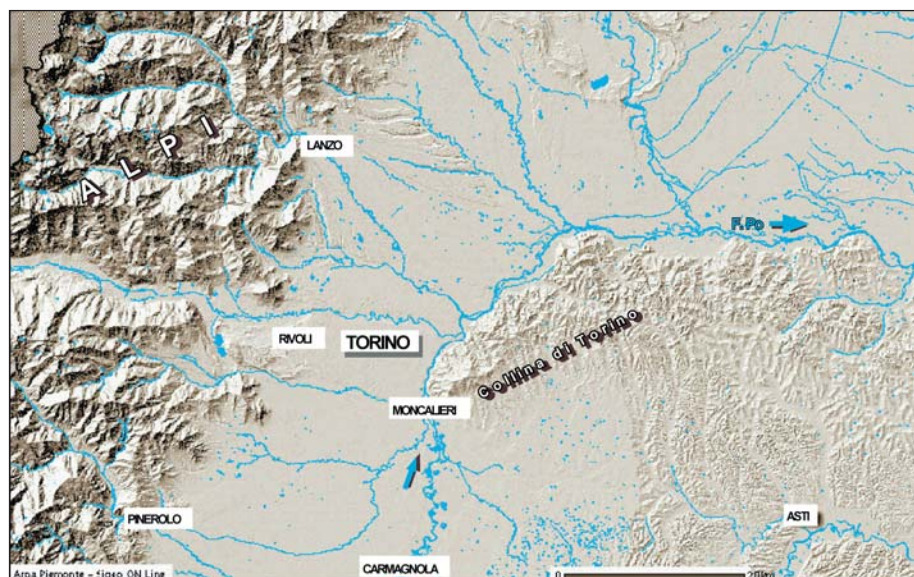
Fig. 3 - Modello Digitale del Terreno del Piemonte centrale: la Collina di Torino, incisa al margine settentrionale dall'attuale F. Po, forma un rilievo che si innalza di circa 500 m sulla pianura, costituita dagli estesi conoidi dei corsi d'acqua alpini (modificato da ARPA Piemonte, SigeoOnline, 2004).
