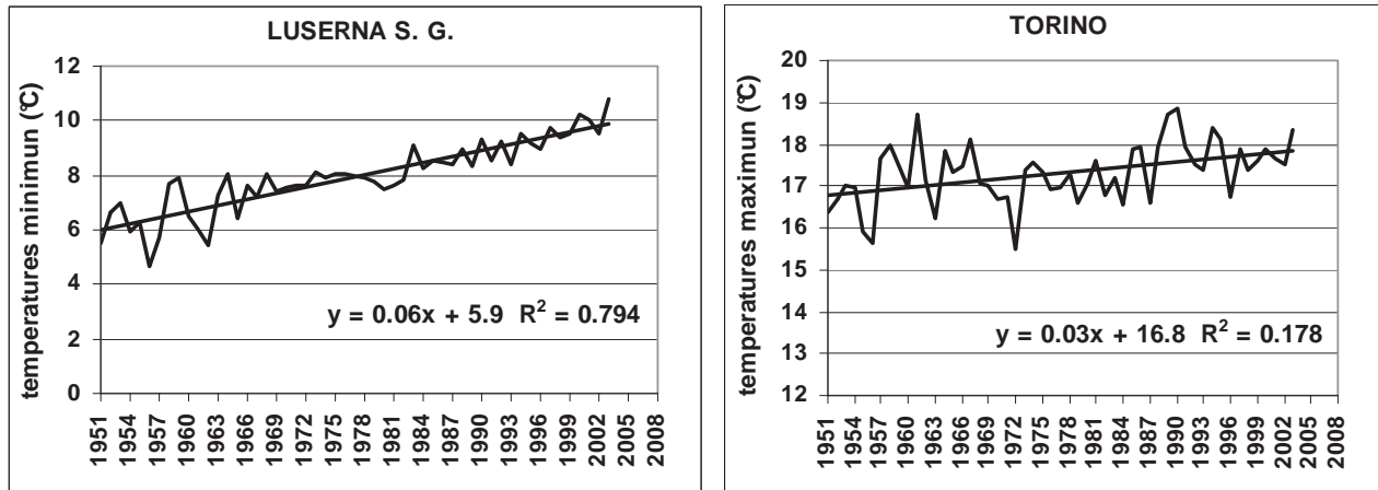
Figure 3. Tendance des températures minimum annuelles calculée dans la localité de Luserna S. G. et tendance des températures maximum annuelles calculée à Turin pour une période de 53 ans, de 1951 à 2003.
