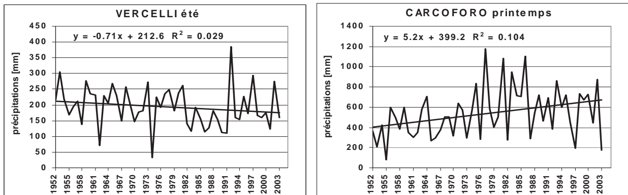
Figure 2. Tendances des précipitations saisonnières calculées dans la localité de Vercelli en été et dans la localité de Carcoforo au printemps pour une période de 52 ans, de 1952 à 2003.
