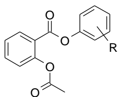
2, NCX4040 R = p-CH 2 ONO 2
