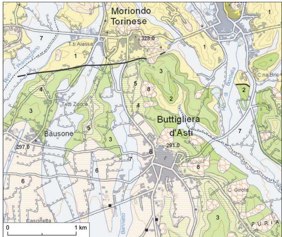
Fig. 7 - La Zona di Faglia di Castelnuovo don Bosco che disloca la successione "villafanchiana". 1: Sabbie di Asti. 2: Silt di San Martino ("Villafanchiano" Auct.). 3: Sabbie di Ferrere ("Villafanchiano" Auct.). 4: Sintema di Morialdo. 5: Sintema di Buttigliera. 6: Sintema di San Giovanni. 7: Sintema di Palazzolo. 8: depositi di frana.
