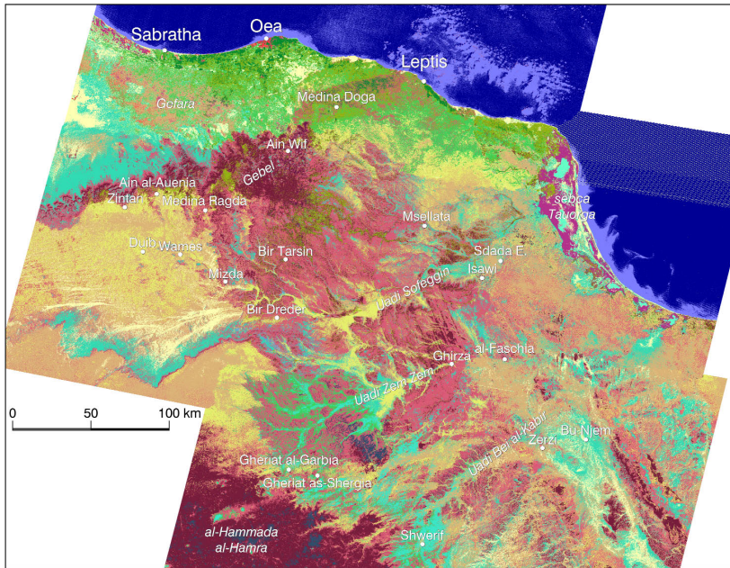
Fig. 1 – Elaborazione di immagini multispettrali Landsat relative alla Tripolitania al fine della ricognizione dei vari tipi di terreno e della copertura vegetale (N. Masturzo 2008).
