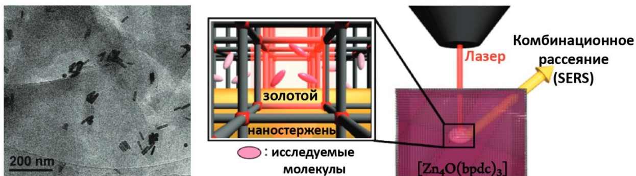
Рис. 7. Синтез [Zn_4O(bpdc)_3] металлоорганической каркасной структуры вокруг золотых наностержней. Справа показано применение полученной структуры для поверхностно-усиленной спектроскопии комбинационного рассеяния света. Рисунок адаптирован из работы [296].
