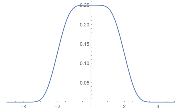
FIGURE 1. The graph of the distribution function g(x) of X . Le graphe de la fonction de distribution g(x) de X .
