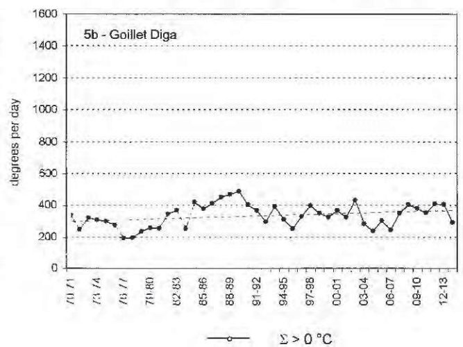
FIG. 4b e 5b - Degrees per day trend of June at Chiotas Diga and Goillet Diga. Andamento dei gradi-giorno di Luglio e Agosto a Chiotas Diga e Goillet Diga.
