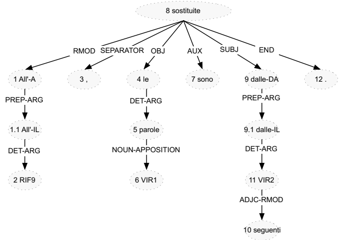
Figure 4: Syntactic analysis of the sentence: All’articolo 40, comma 1, della legge 28 dicembre 2005, n. 262, le parole “sei mesi” sono sostituite dalle seguenti: “dodici mesi” [At the article 40, comma 1 of the law December 28, 2005 number 262, the words “six monts” are substituted by the following: “twelve monts”].
