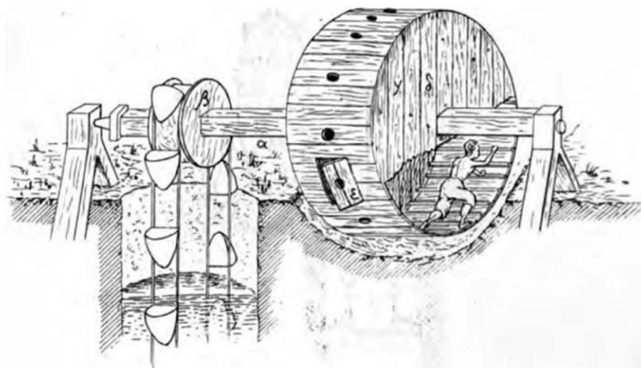
Fig. 1. Ruota idraulica a catena di secchi con attivazione a passo umano (immagine tratta da CARRA DE VAUX, Le livre des appareils , p. 226)
