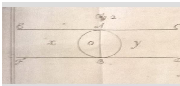
Figura 2 – distanza costante tra due rette parallele
