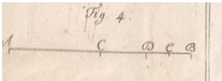
Figura 4 – segmento unitario dicotomizzato
