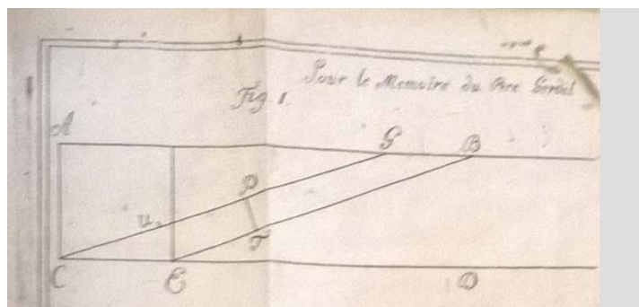
Figura 1 – prolungamento all'infinito delle rette parallele
