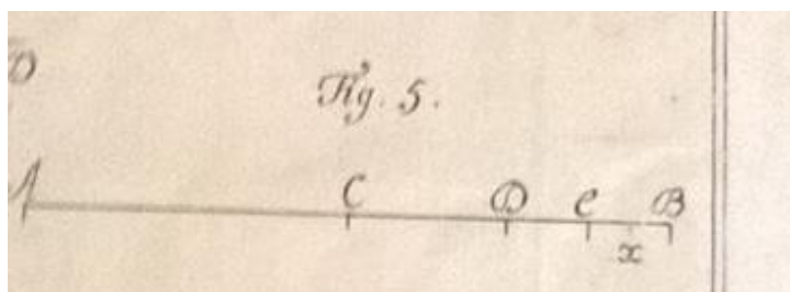
Figura 5 – segmento unitario dicotomizzato con ultimo termine della suddivisione non nullo
